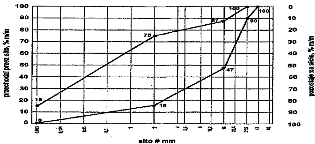
Rys. 5. Krzywe graniczne uziarnienia mieszanki kruszyw 0/31,5 mm do warstwy podłoża ulepszonego
