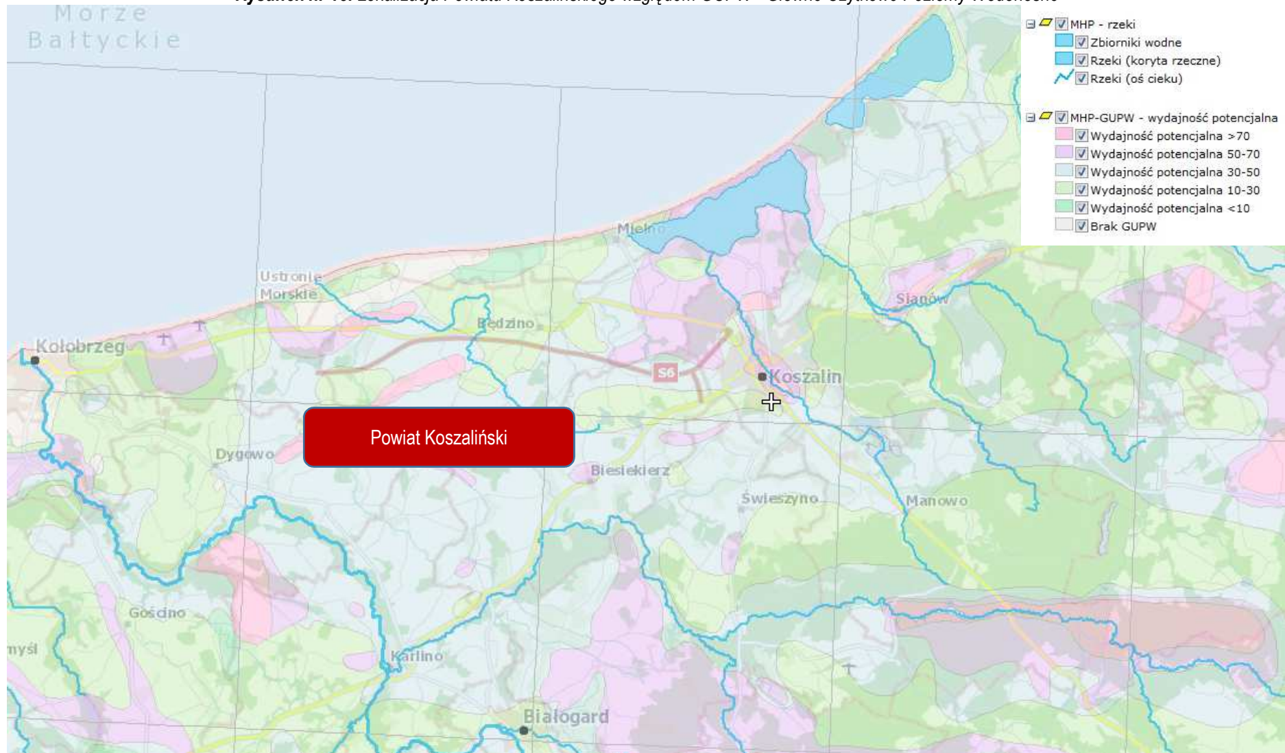
Rysunek nr 13. Lokalizacja Powiatu Koszalińskiego względem GUPW - Główne Użytkowe Poziomy Wodonośne
